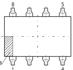
Схемы расположения выводов
